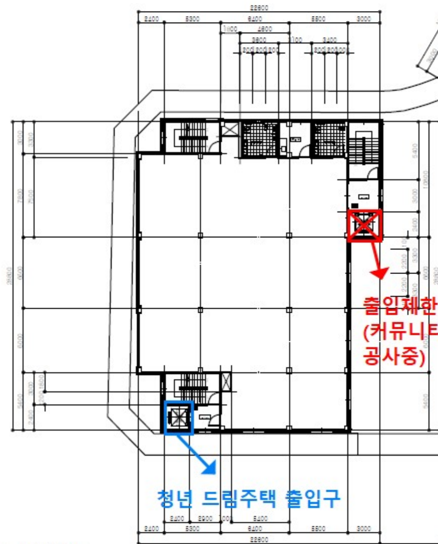
A동 2층 평면도 scale : 1/ 300
